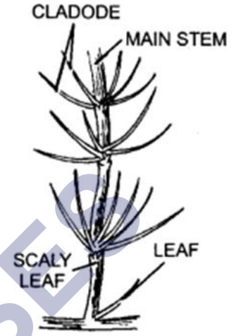
सतावर में पर्णाभ-पर्व।
