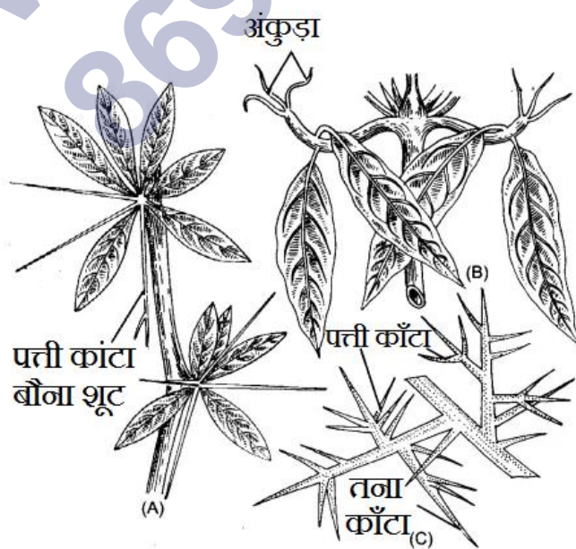
पर्णकंटक : (A) बारबेरी, (B) बिगोनिया तथा (C) यूलेक्स में।
